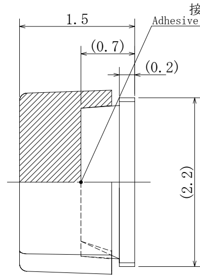
カソードマーク Cathode Mark (C0.25)
